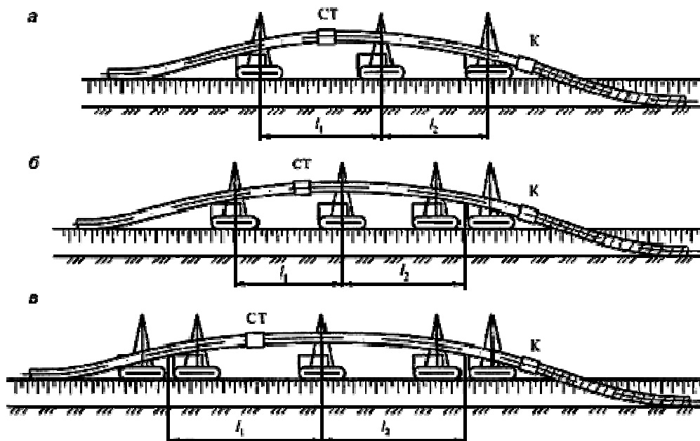
Рисунок 21 - Совмещенный способ изоляции и укладки газопровода диаметром: а - 500-800 мм; б - 800-1000 мм; в - св. 1000 мм при использовании комбайна. Возможно также совмещение операций по изоляции стыков и укладке газопровода.
