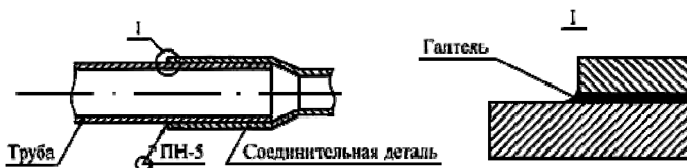
Рисунок 16 - Схема паяного соединения
