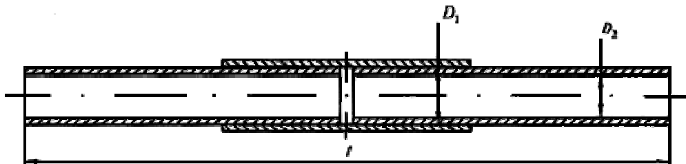
Рисунок 8 - Допускное соединение
