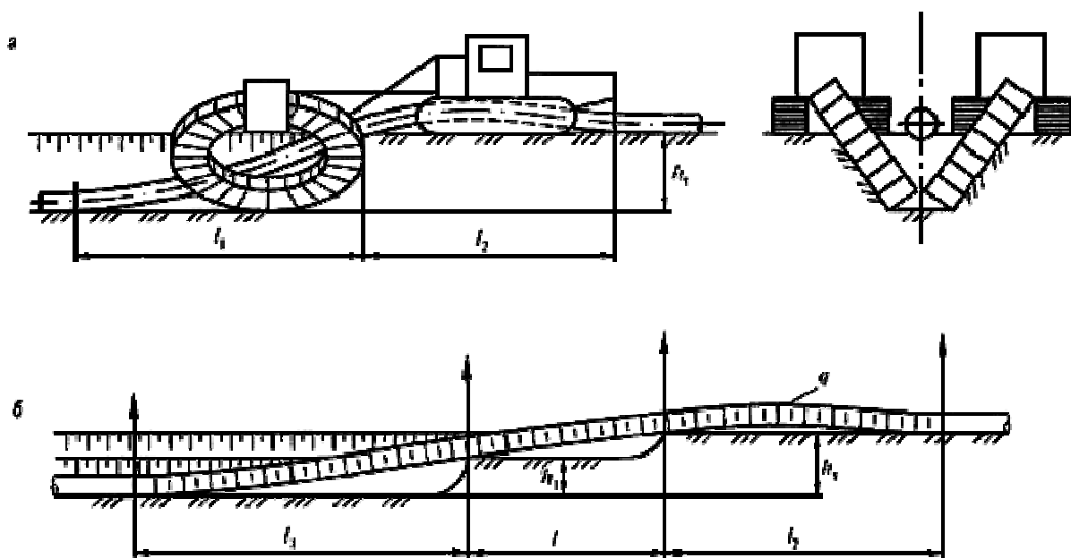
Рисунок 23 - Укладка газопровода методом "подкопа"
